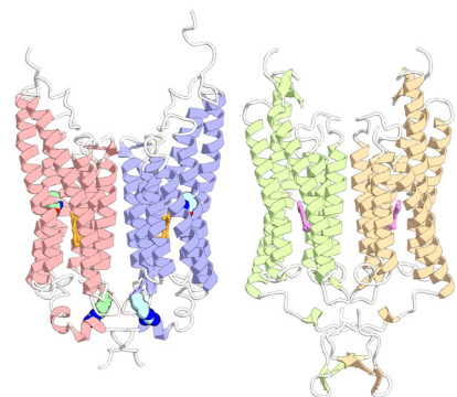
(左)天然型、(右)人工型の陰イオンチャンネルロドプシン結晶構造 (Kato et al., Nature , 2018)
